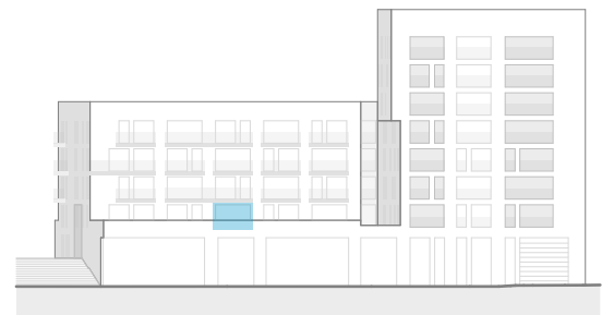
ANSICHT OST
