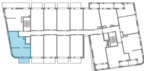
GESCHOSSPLANUNG 4.OG
